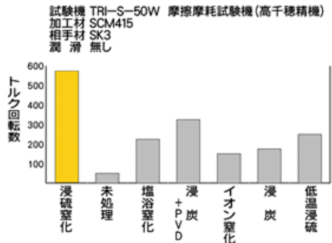
図-1 各種表面改質の妬き付け試験比較表
