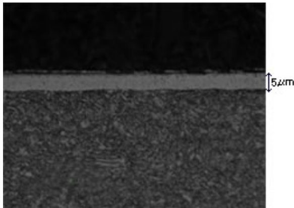
SCM415浸炭品に処理
